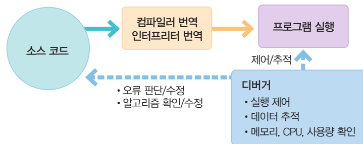
▲ [그림 I-16] 디버거의 제어/추적 기능
