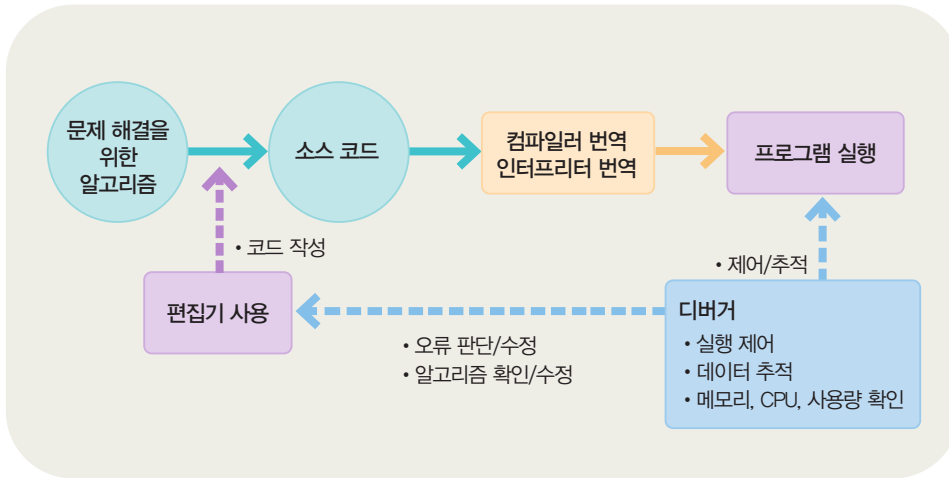
▲ [그림 I-17] 통합 개발 환경
